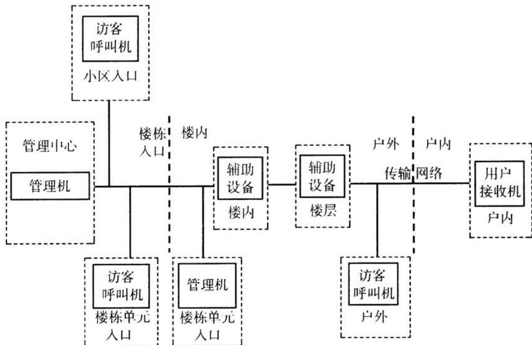
图 6 楼寓对讲系统应用构成示意图
