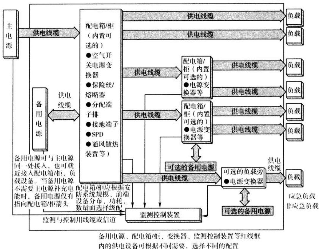
图7 安全防范系统供电系统构成示意图
