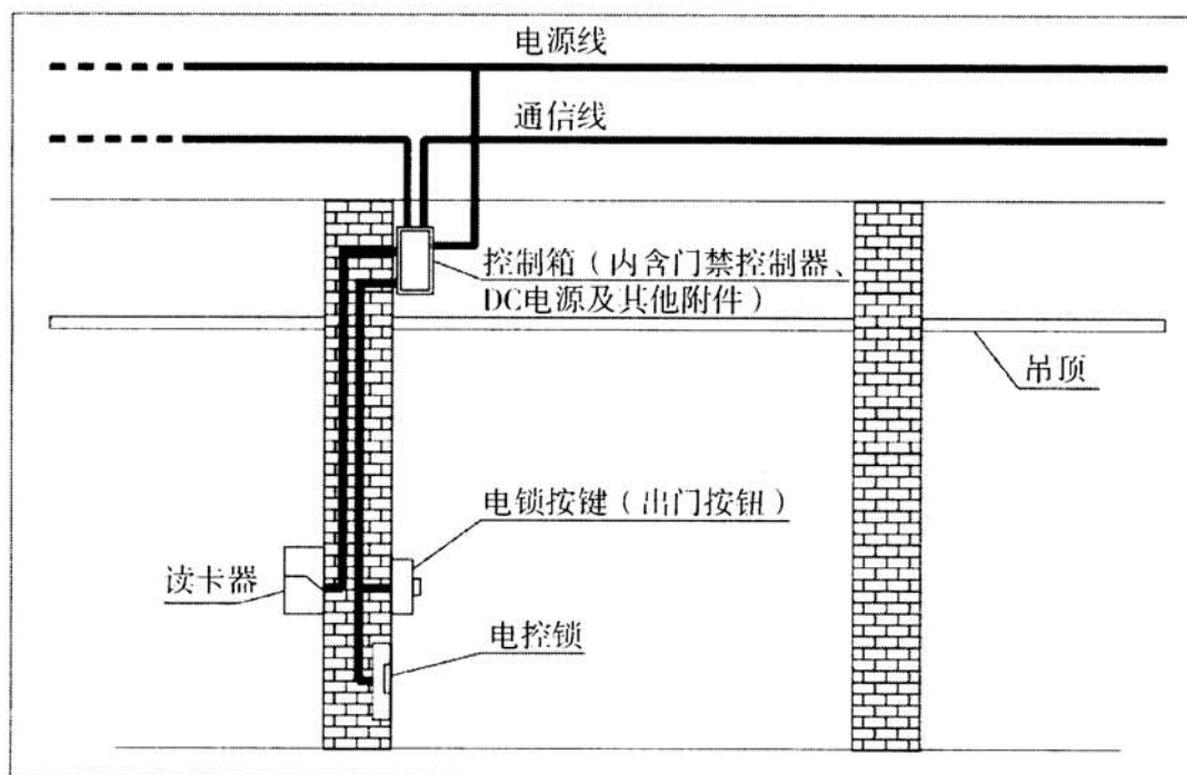
图 8 出入口控制设备安装管线示意图
