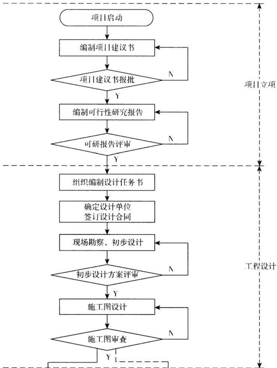
图 2 安全防范工程建设程序示意图
