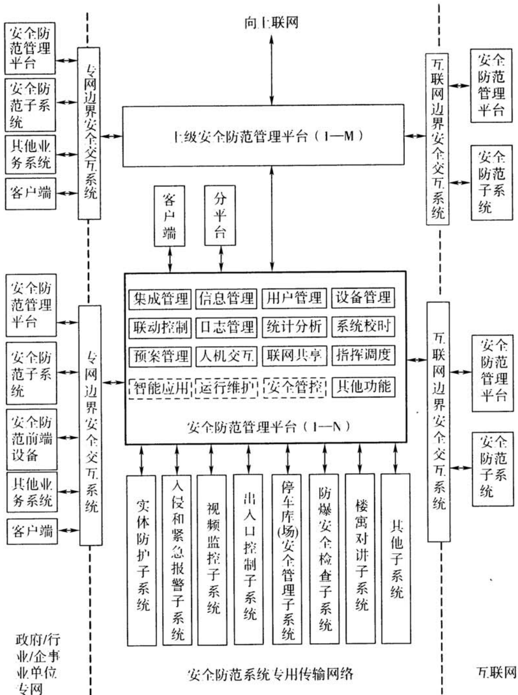
图 1 安全防范系统集成联网架构图
