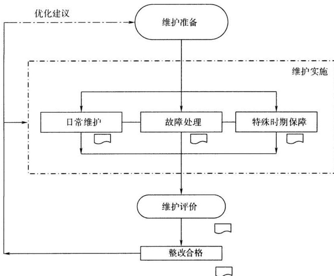
图 10 安全防范系统维护工作程序
