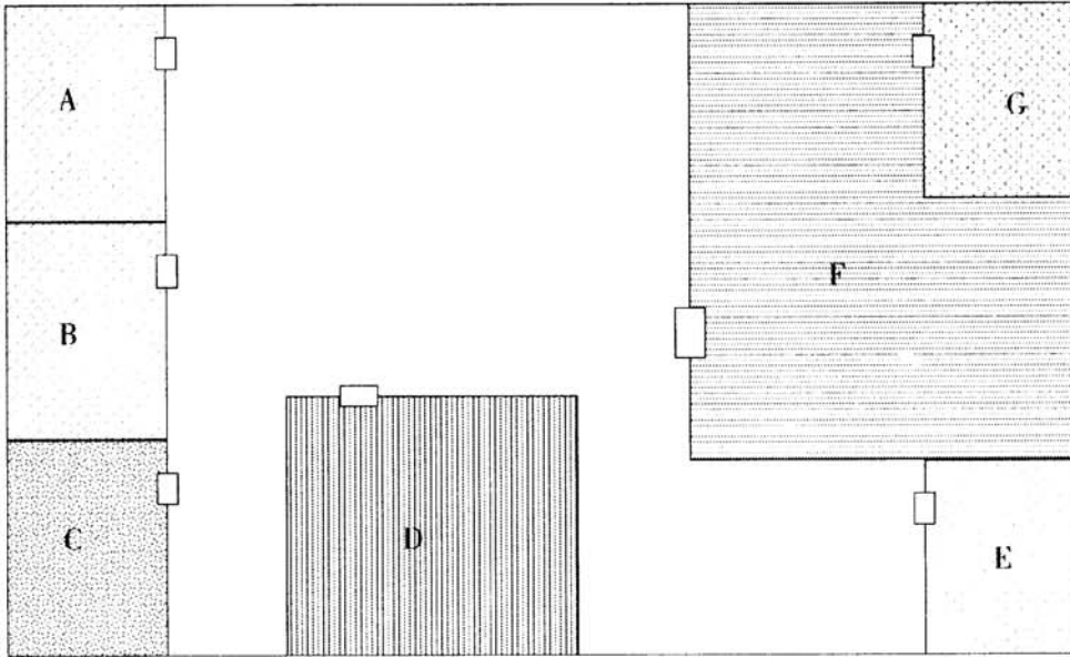
图3 出入口控制系统受控区示意图
