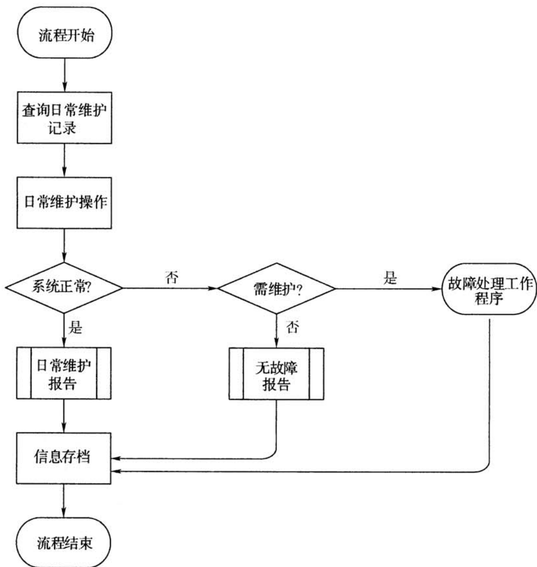
图 11 安全防范系统日常维护工作程序
