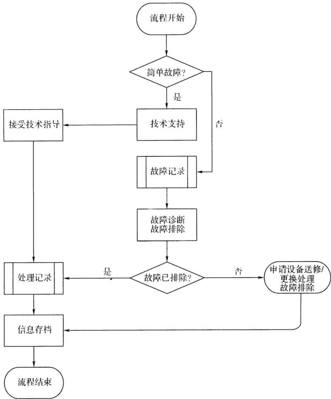
图 12 安全防范系统故障处理工作程序
