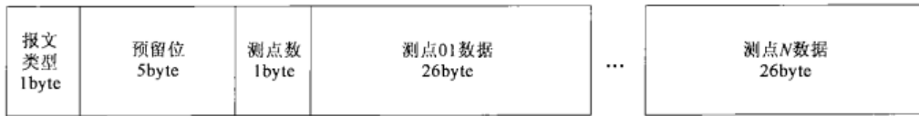
图 D.2 GNSS 报文协议结构组成
