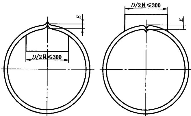
图4 筒体纵焊缝棱角高度
