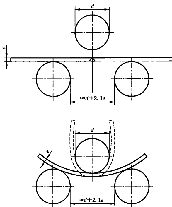
图 7 对接接头弯曲试验
