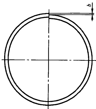
图3 筒体纵焊缝对口错边量
