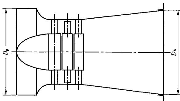
图9 集风器的进口直径 D_k
