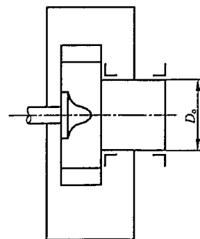
图10 筒形进口直径 D_o
