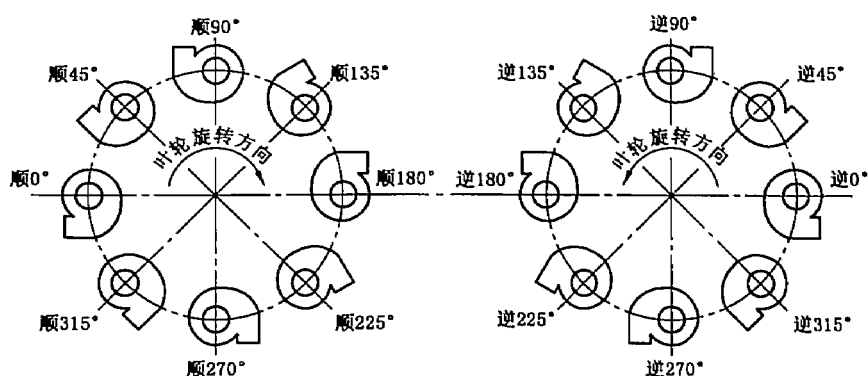
图7 离心风机出气口的安装位置
