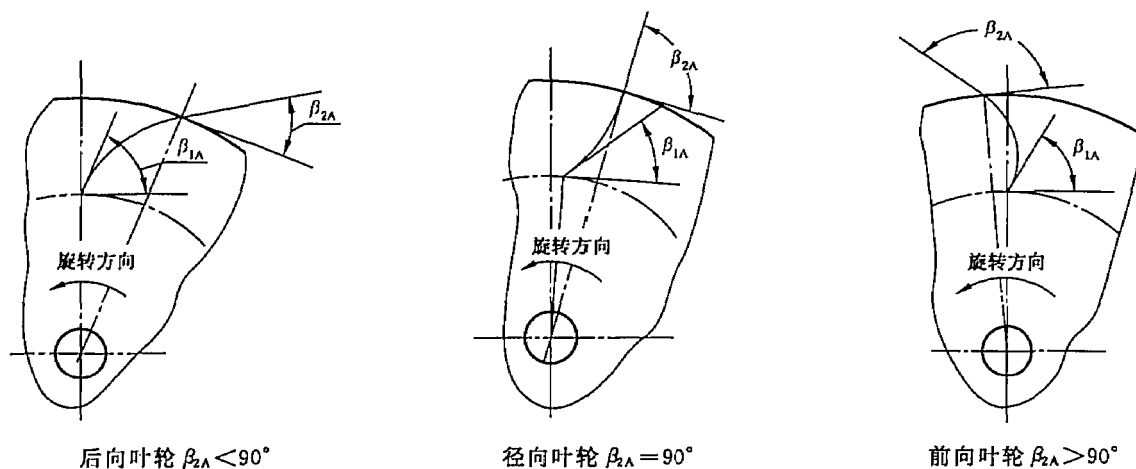
图3 离心通风机叶轮叶片进、出口安装角( \beta_{1A} 、 \beta_{2A} )的表示方法
