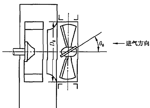
图4 轴向进气
