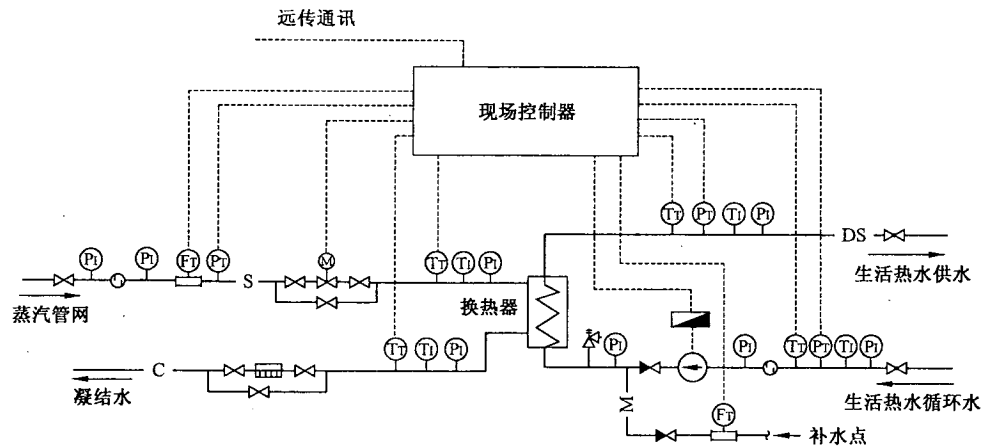
图 A.3 汽-水生活热水换热机组工艺控制流程示意图
