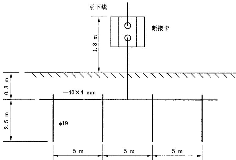
图 B.1 单独热力站接地图
