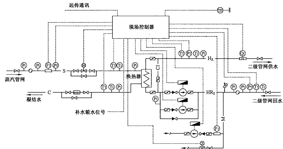
图 A.1 汽-水采暖换热机组工艺控制流程示意图
