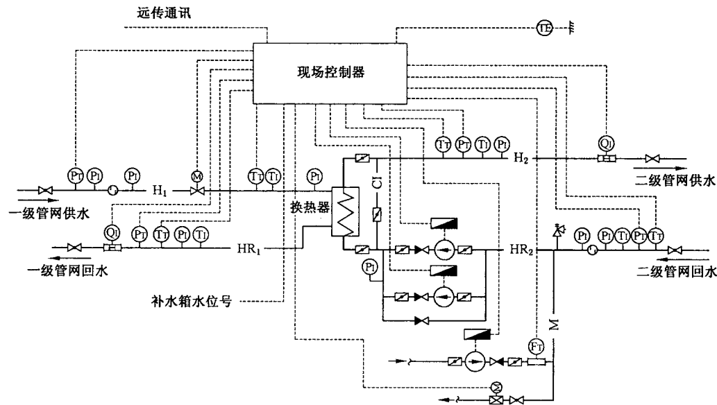
图 A.2 水-水采暖换热机组工艺控制流程示意图
