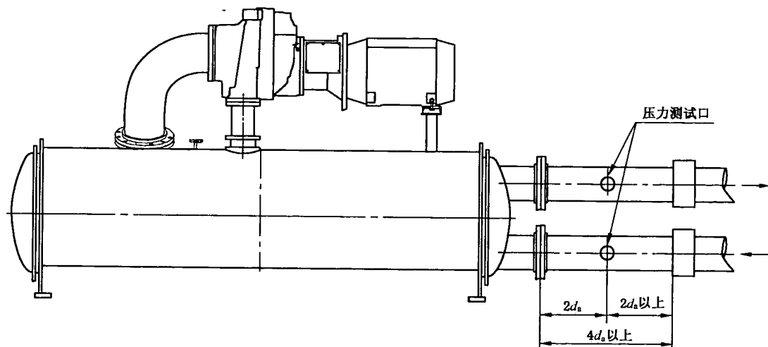
图 B.3 压力测试管
