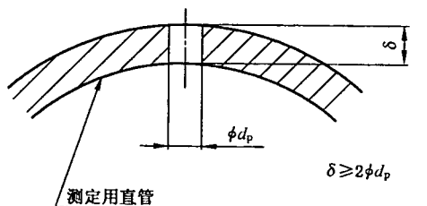
图 B.4 压力测试孔
