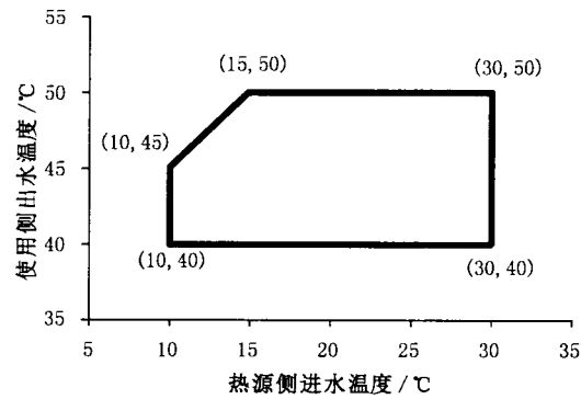
图 B.8 地表水式机组制热运行变工况范围
