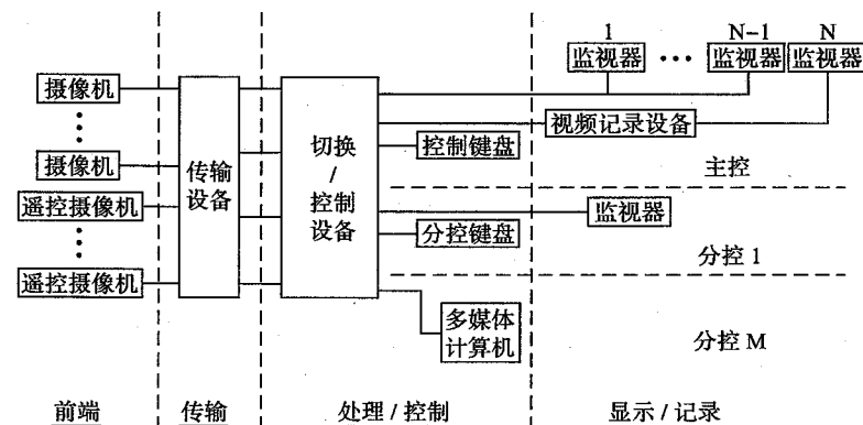
图 4.0.2-3 矩阵切换模式
