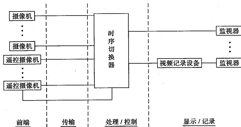
图 4.0.2-2 时序切换模式
