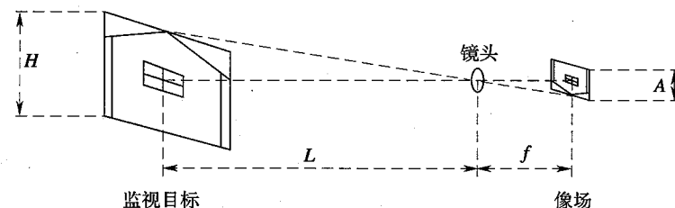
图 6.0.2 光学成像关系图
