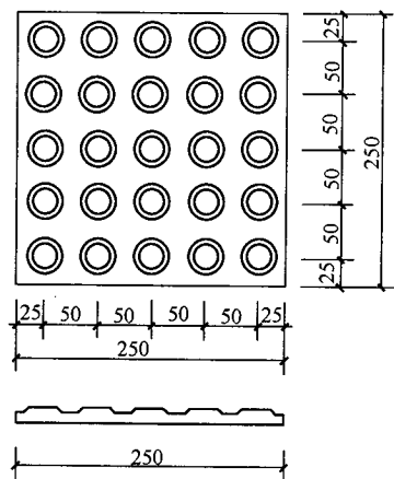
图 3-4 提示盲道
