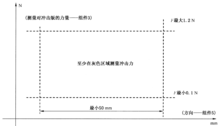
图 11 冲击力分布
