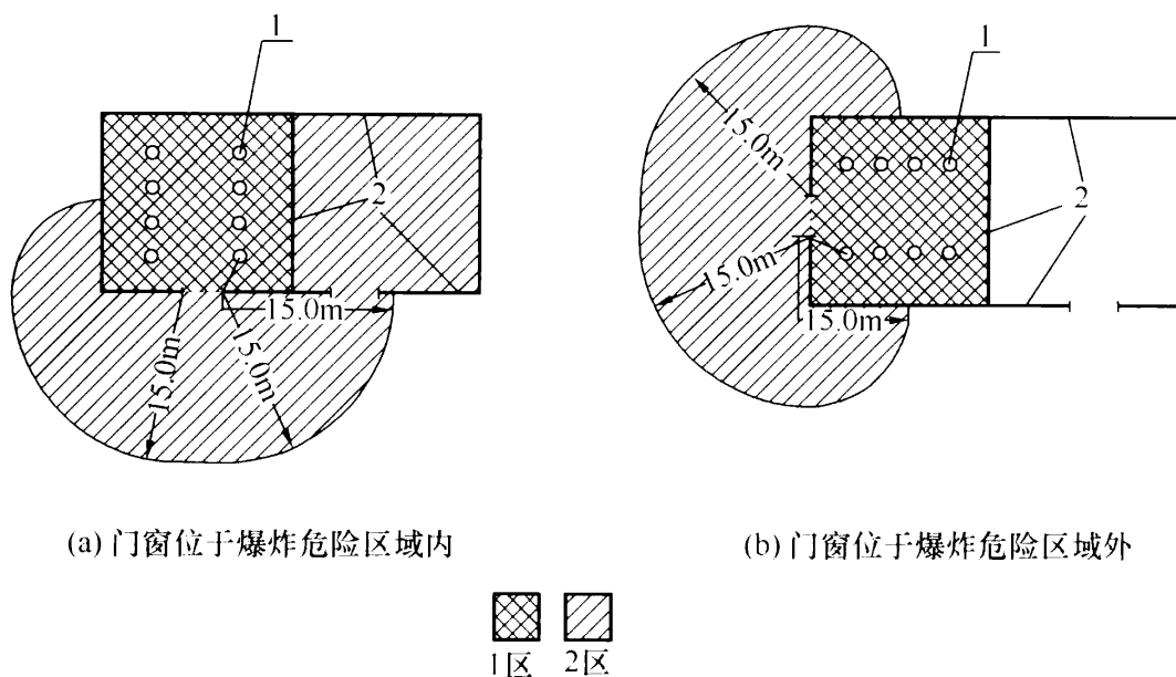
图 A.0.5 无释放源的建筑物与通风不良且有二级释放源的建筑物相邻，当采用不燃烧体实体墙隔开时，其爆炸危险区域和范围划分图
