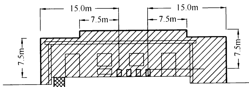
A-A 视图
