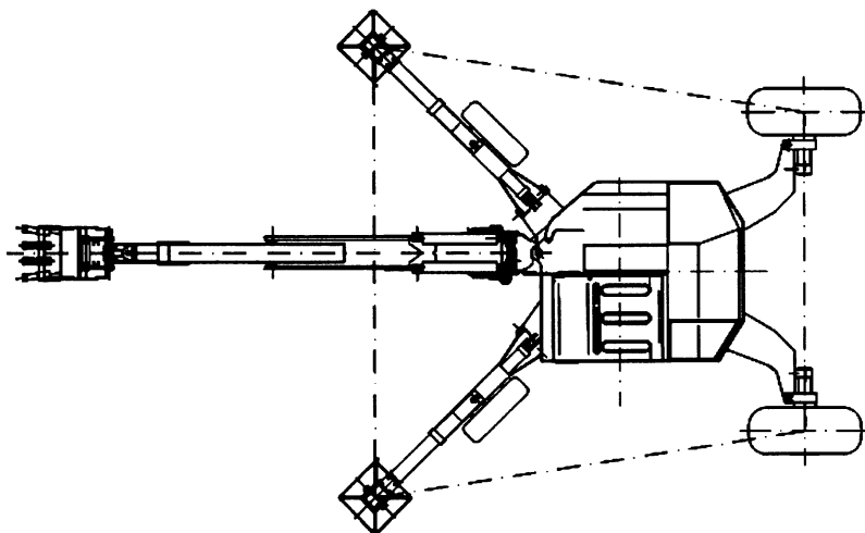
图 1 步履式挖掘机的倾翻线
