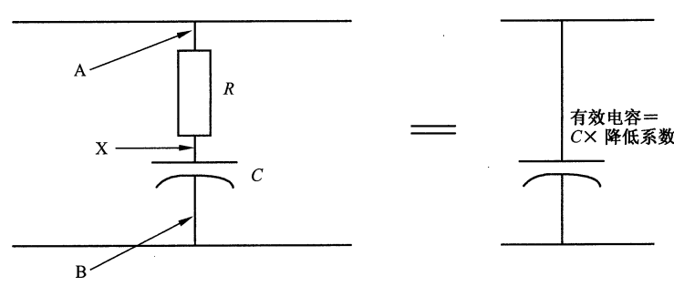
图 A.9 等效电容
