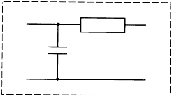
d) 本安电路中熔断器的保护
