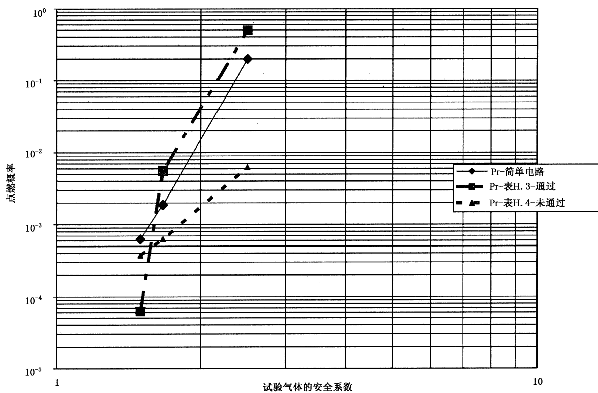
图 H.1 安全系数与点燃概率
