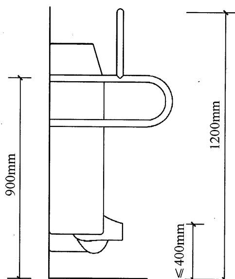
图 7 无障碍小便器安全抓杆侧立面图
