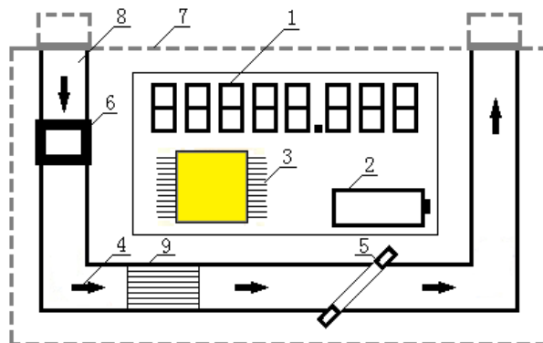
图2 家用超声波燃气表一般结构示意图
